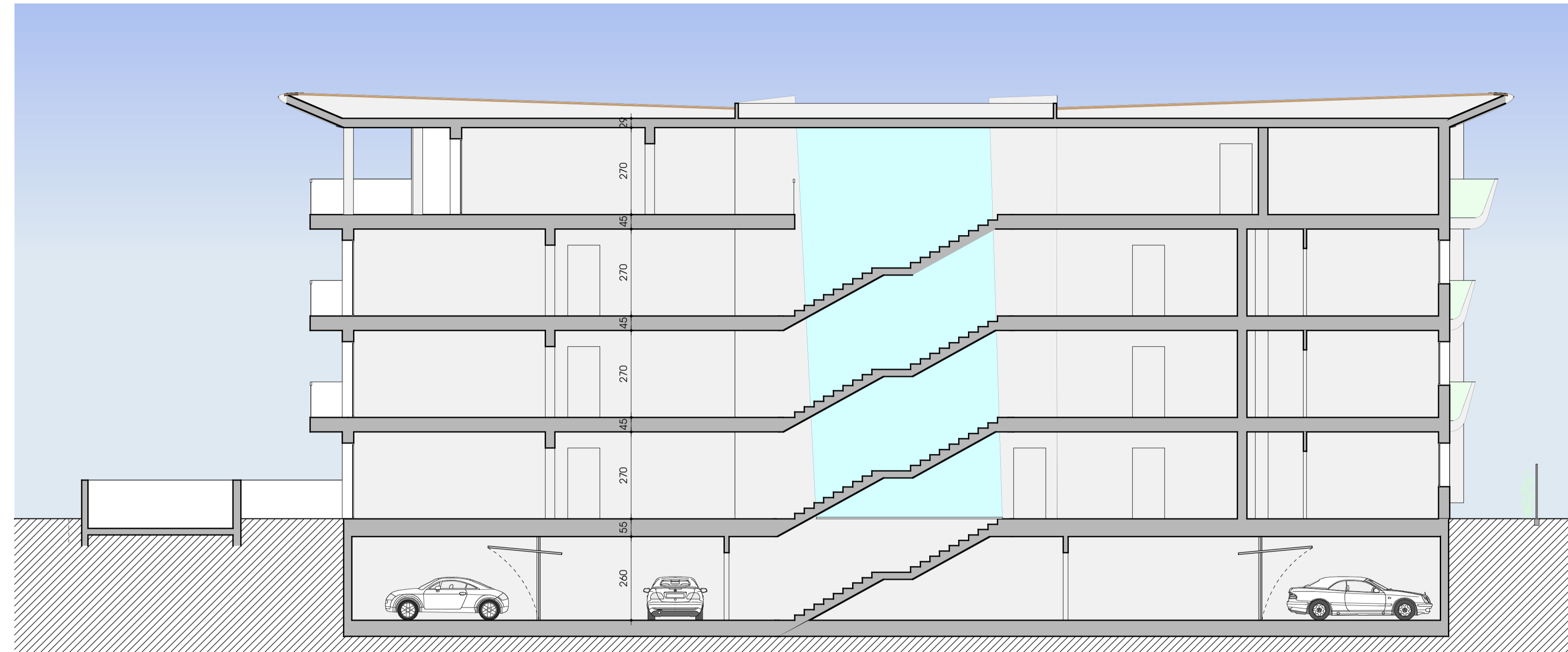
SEZIONE LONGITUDINALE
